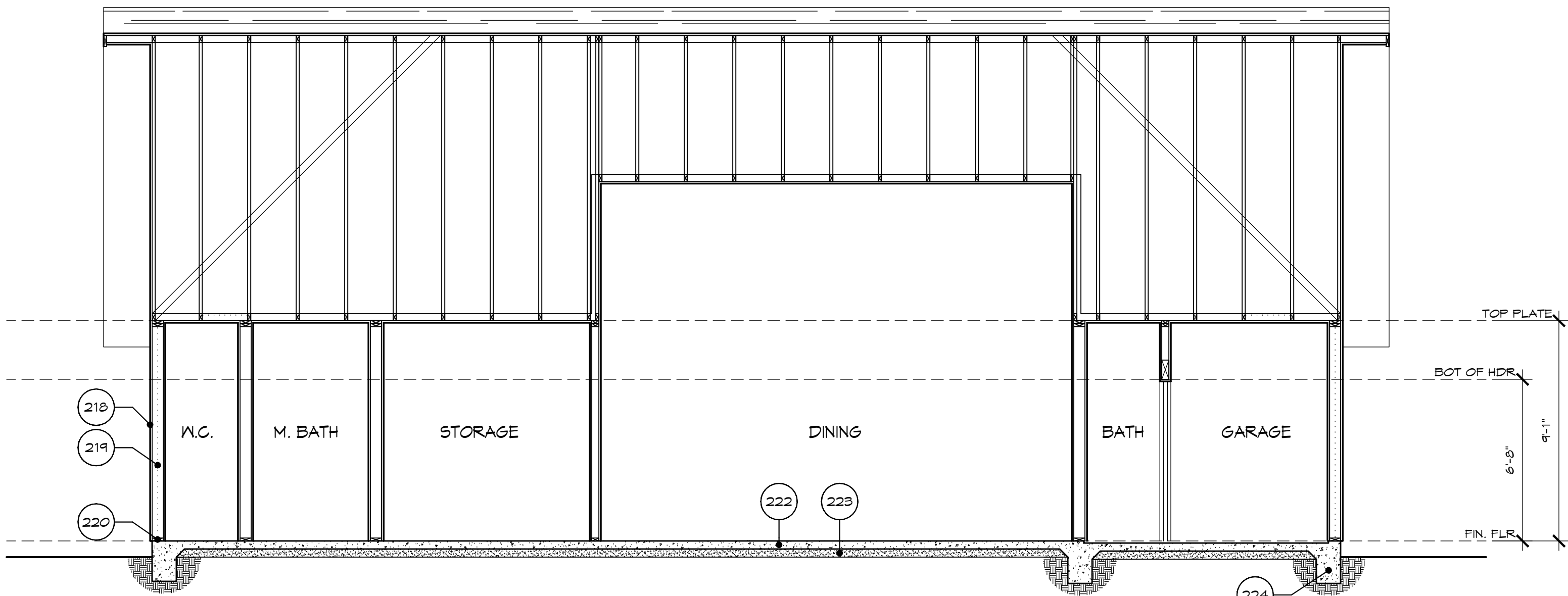
SECTION 'B'
