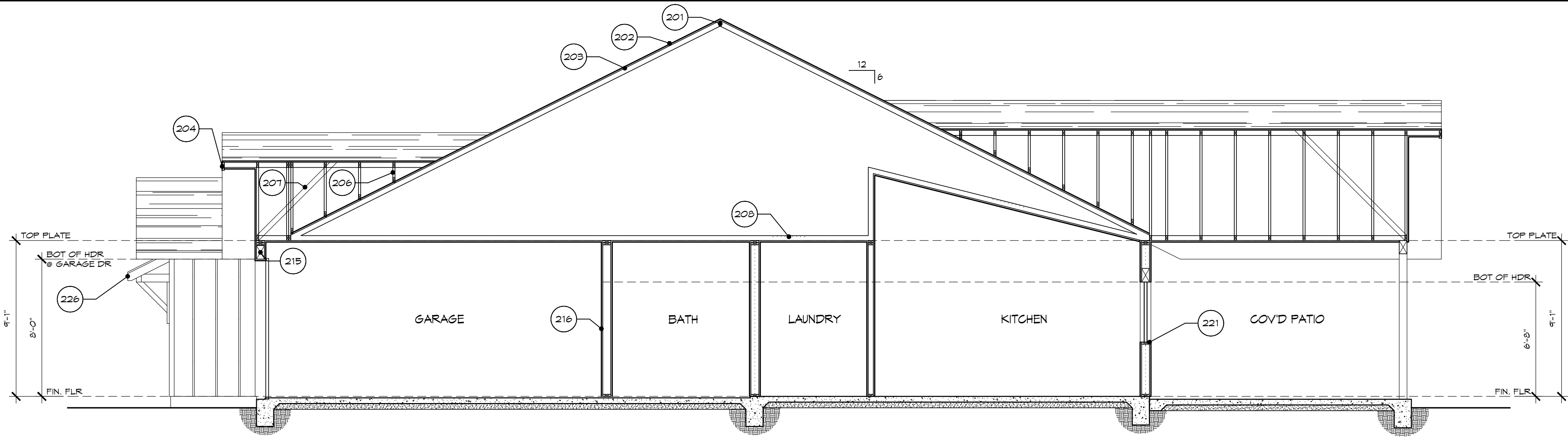
SECTION 'B'
