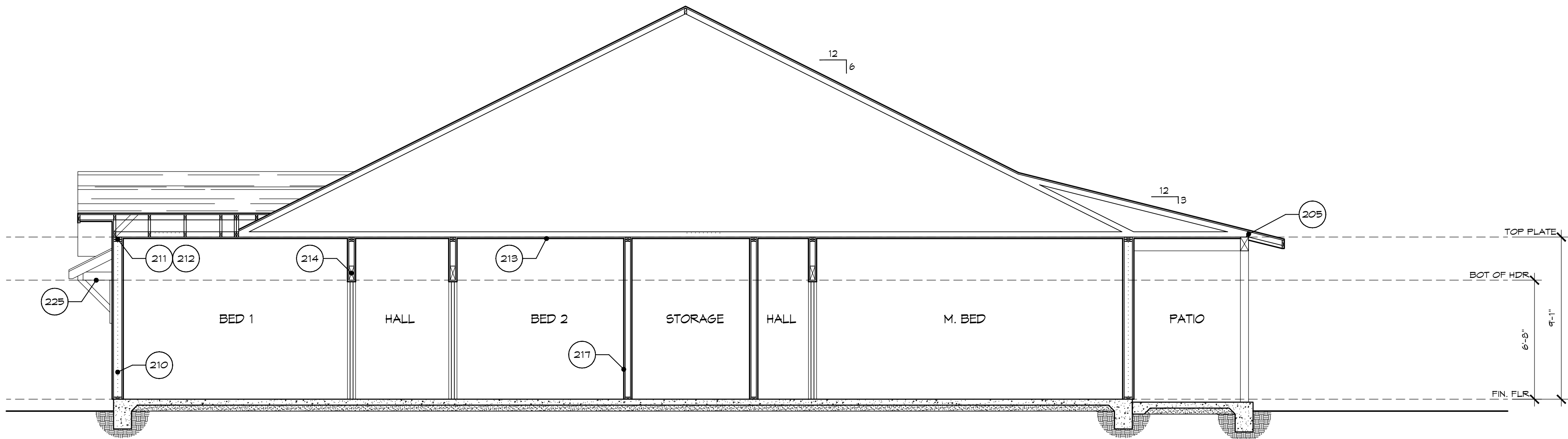
SECTION 'B'
